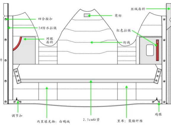
防寒服内里结构图：
