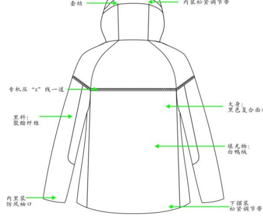
防寒服背面结构图：
