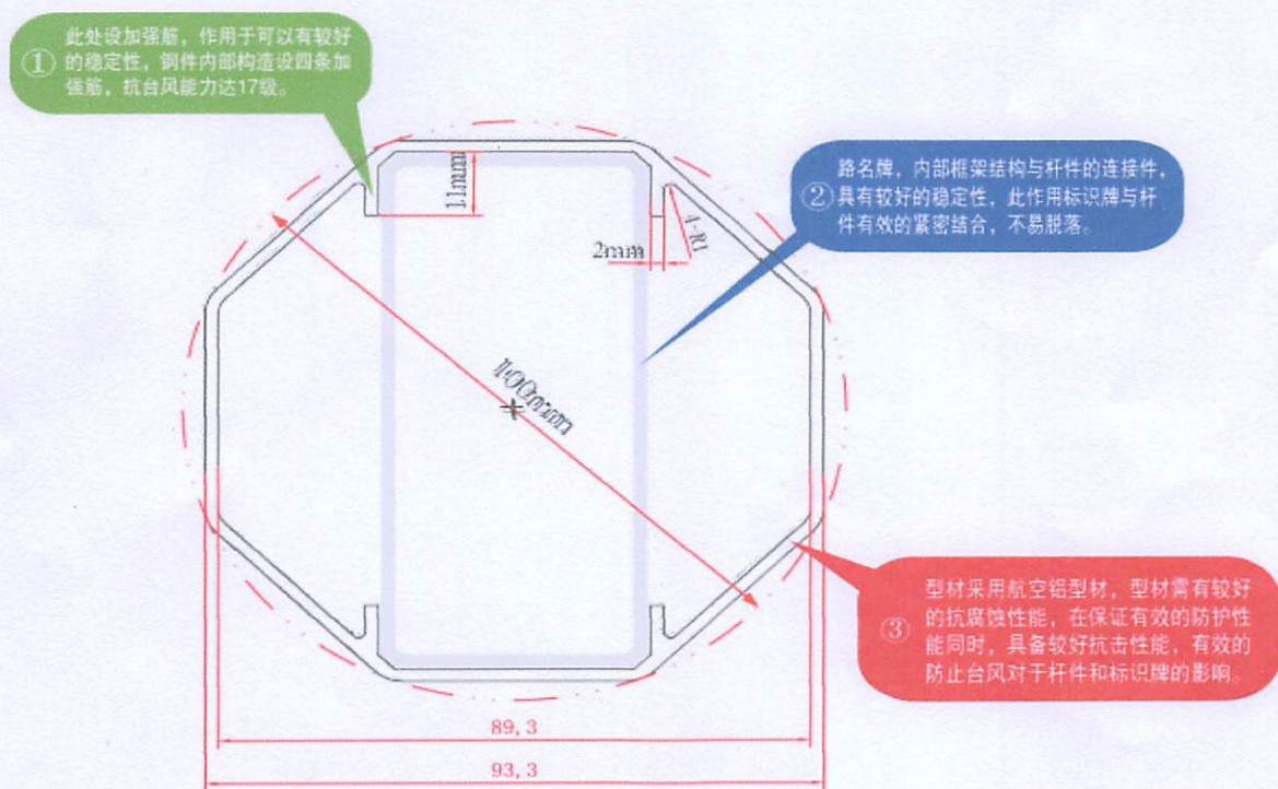
铝型材料管(八角型)结构图
