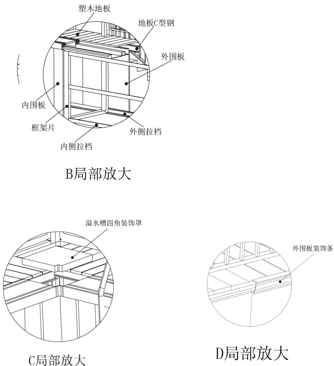
图 1 产品结构示意图
