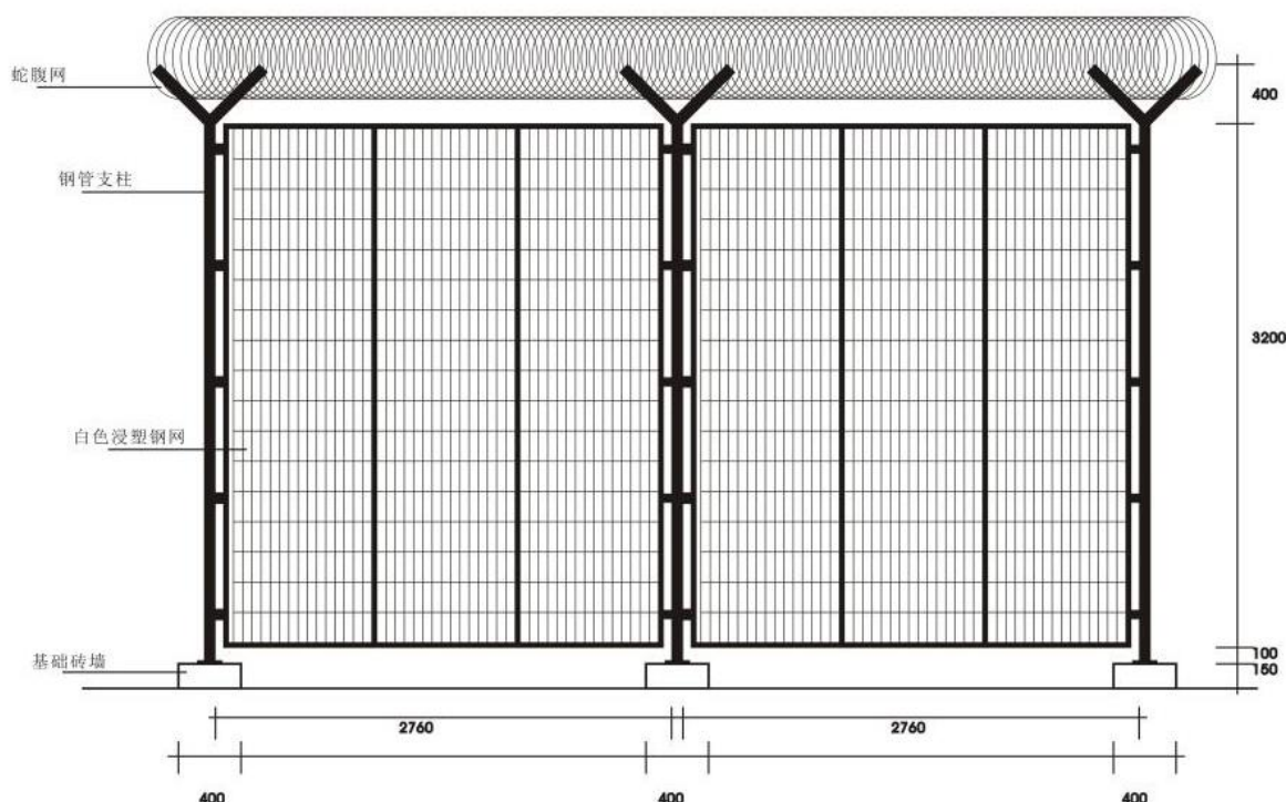
三江监狱监仓内警戒区钢网墙工程示意图 设计说明
