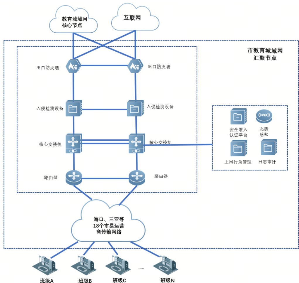
图 1-1儋州市教育城域网网络架构图
