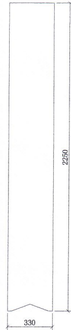
不锈钢碗架侧立面图
