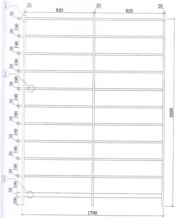
不锈钢碗架正立面图
