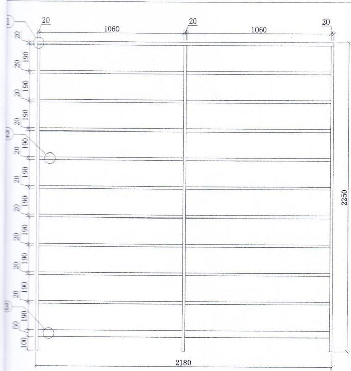
不锈钢碗架正立面图
